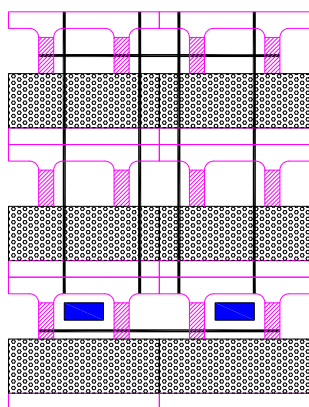
PACCO di BLOCCHI su BANCALE "BLOCCO CORREA - ANGOLO A PIACERE - ELEMENTI SOLAIO"
