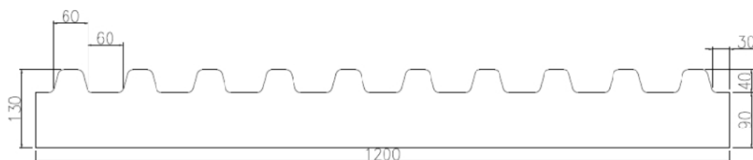
Pannello fonoassorbente in legno-cemento Isotex S 13
