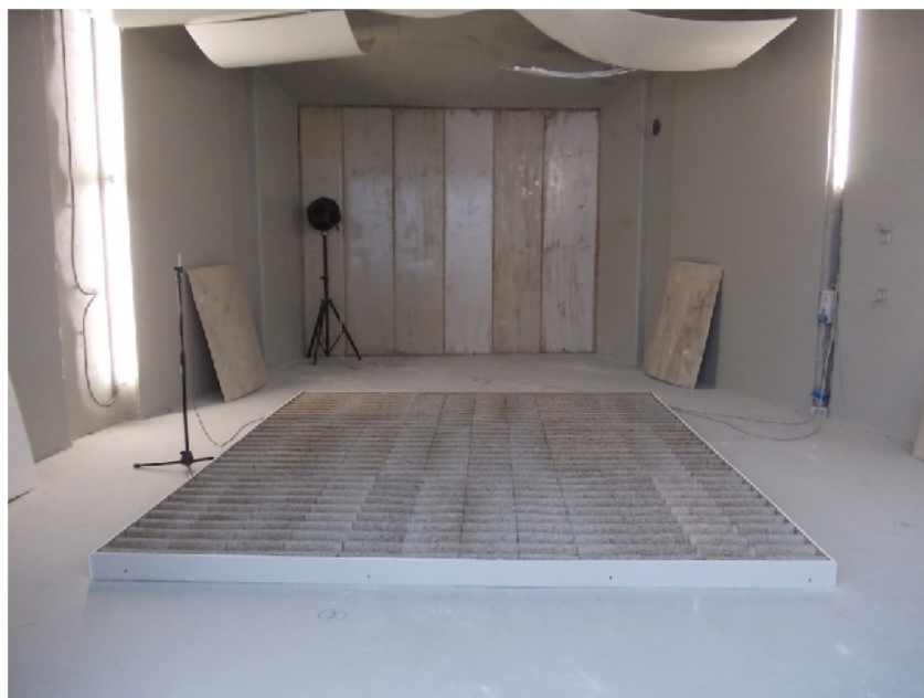
Figura 1. Campione installato nella camera riverberante
