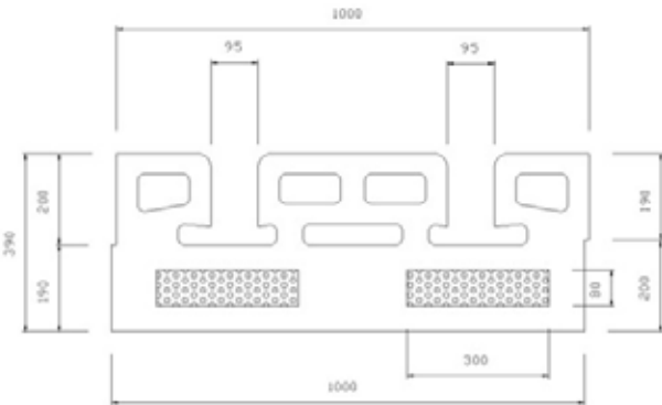
Solaio S39
