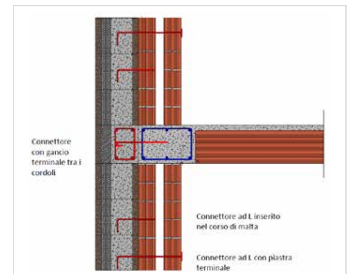
Posizionamento dei connettori nelle travi fondazione
