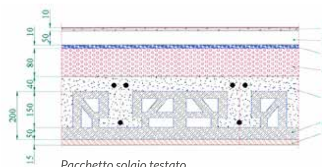
Pacchetto solaio testato
