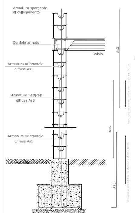
Blocco HDIII 38/14 con grafite Neopor® BMBcert di BASF per pareti portanti esterne
